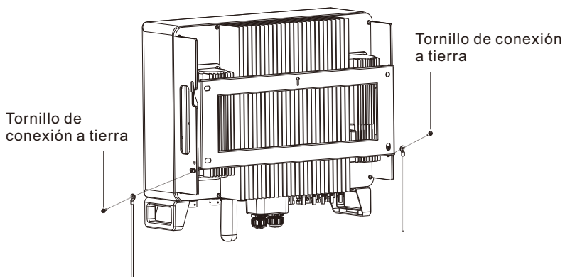
Figura 4.5 Conexión del conductor de tierra externo
