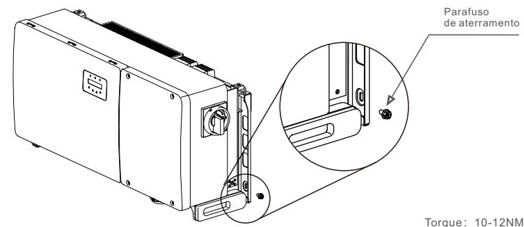
Figura 3.17 Cabo fixo
