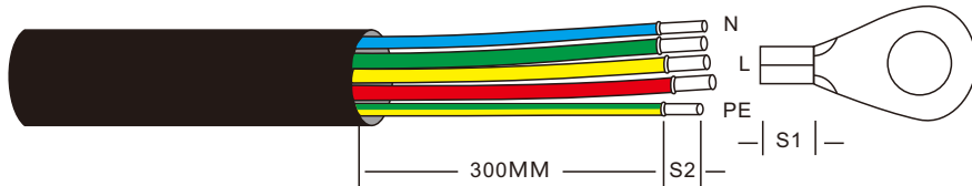
Figura 3.24 Descascar o cabo AC
