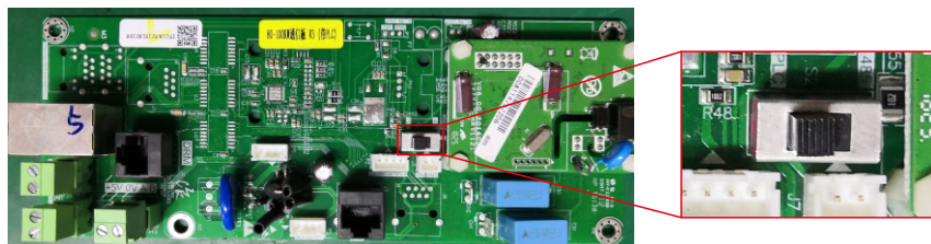
Figura 4.7 Interruptor entre PLC e Rs485
