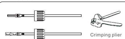
Figura 3.20 Prenda o pino de contato ao fio
