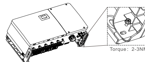
Figura 3.8 Fixe o inversor
