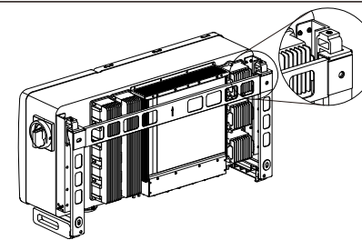
Figura 3.7 Instalação do inversor
