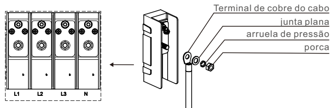
Figura 3.25 Terminal de transferência de cobre-alumínio
