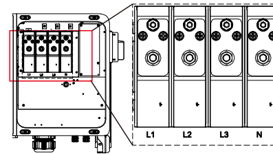
Figura 3.27 Fiação com neutro
