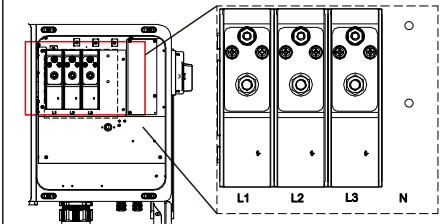
Figura 3.28 Fiação sem neutro
