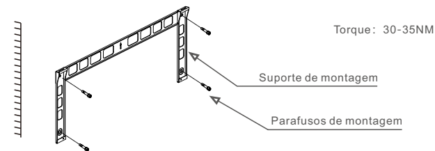
Figura 3.6 Montagem do inversor na parede
