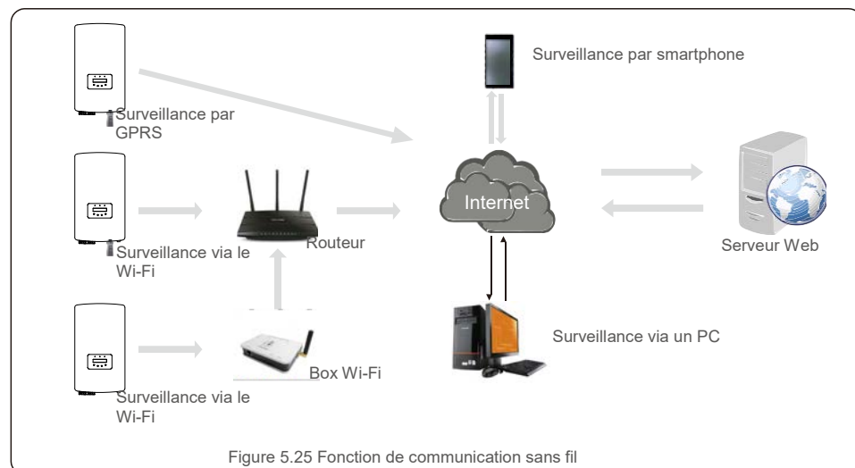
Figure 5.25 Fonction de communication sans fil
