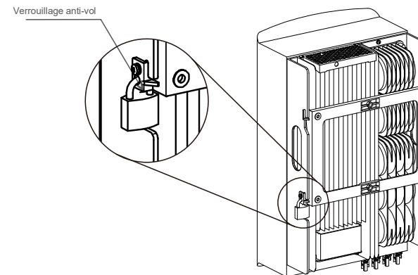
Figure 5.7 Installer le verrou de sécurité
