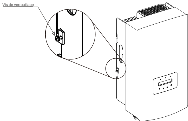
Figure 5.6 Fixation de l'onduleur
