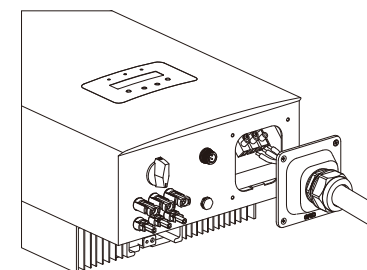
▲ Hình 4.17 Đấu nối cáp với cực nối AC
