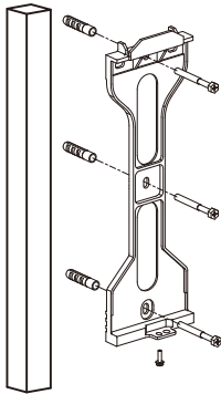
▲ Hình 4.5 Cách gắn biến tần lên cột
