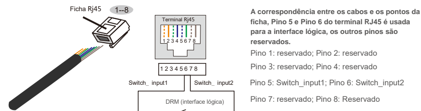
Figura 5.26 Retire a camada de isolamento e ligue à ficha RJ45
