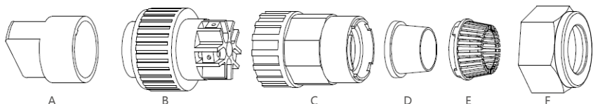
Figura 5.19 Connettore CA
