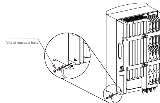
Figura 5.10 Cavo installato
