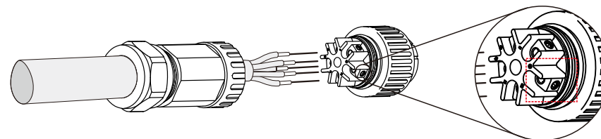
Figura 5.22 Cavo collegato
