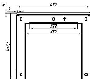
Figura 3.6 Montagem do inversor na parede
