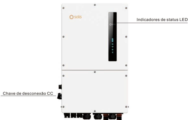
Figura 1.1 Vista frontal
