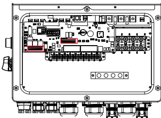
Figura 3.21 Terminais de comunicação
