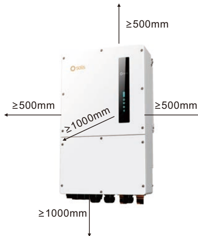
Figura 3.5 Distâncias para montagem do inversor
